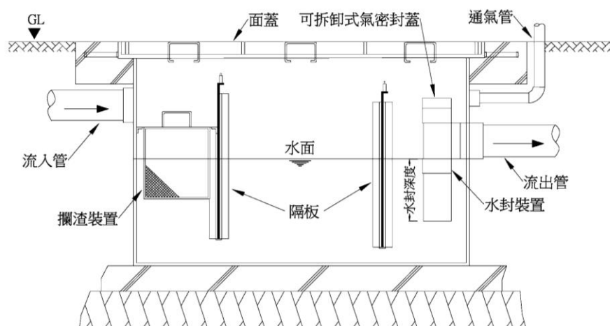
圖4-20 工廠製造的油脂截留器參考圖例
