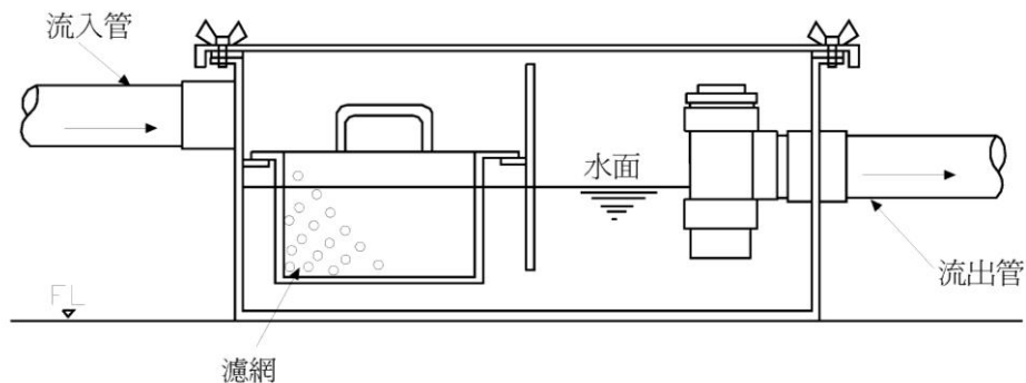
圖4-24 固體物截留器參考圖例
