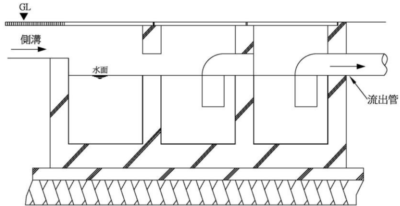
圖4-21 油水分離器參考圖例
